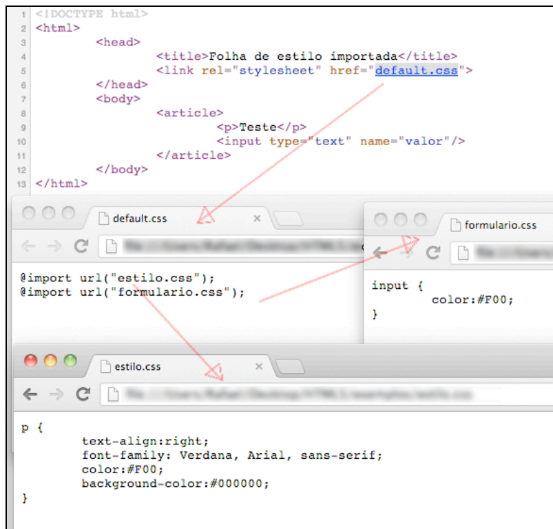
Figura 11 - Tag @import
